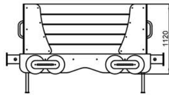
811025 Togvogn, kul HPL L2550xB1350xH1120 mm
